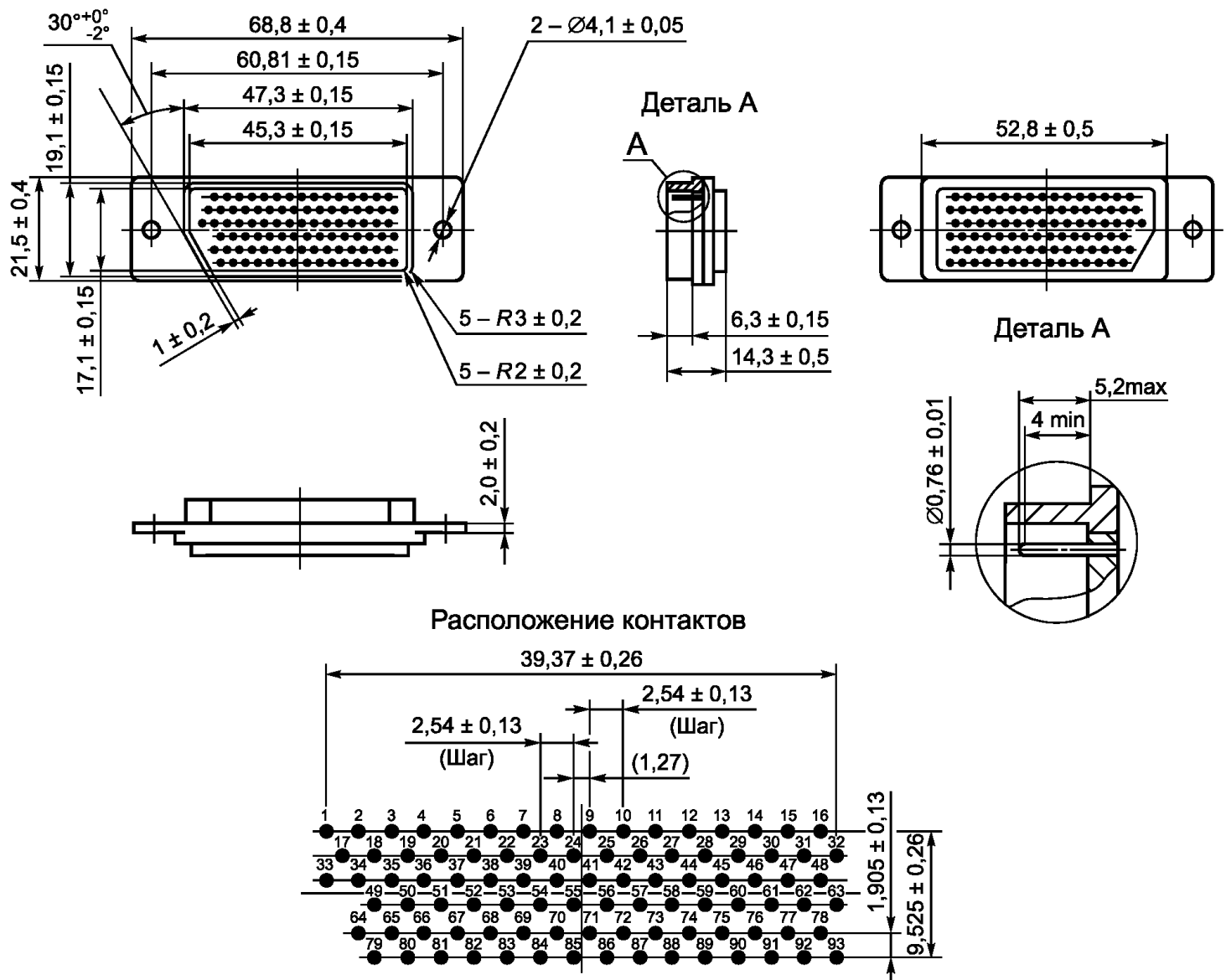
Рисунок 10 — 93-й контактный разъем (вилка)
