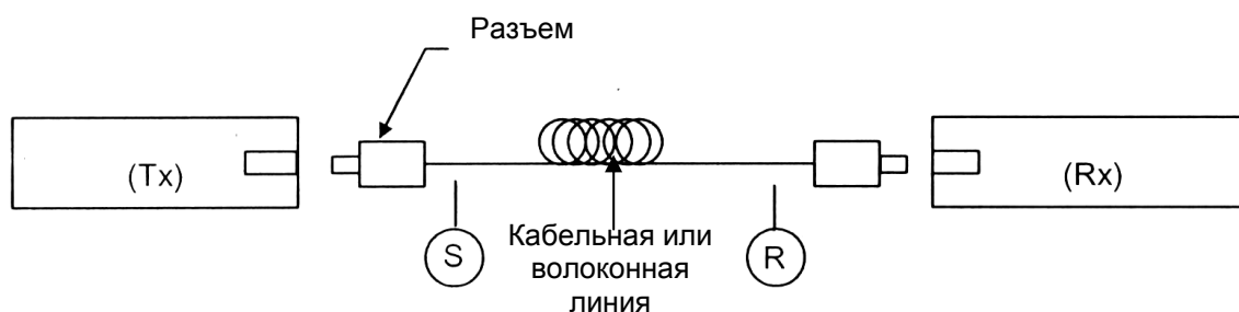
Рисунок 18 - Опорные точки последовательной линии слоя L0
