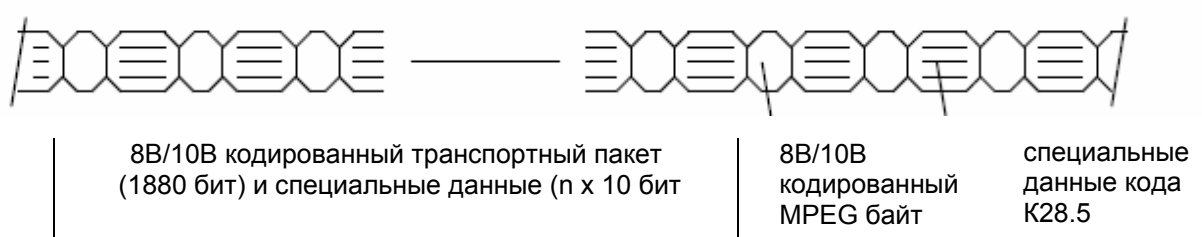
Рисунок 22- Формат передачи отдельных байт
