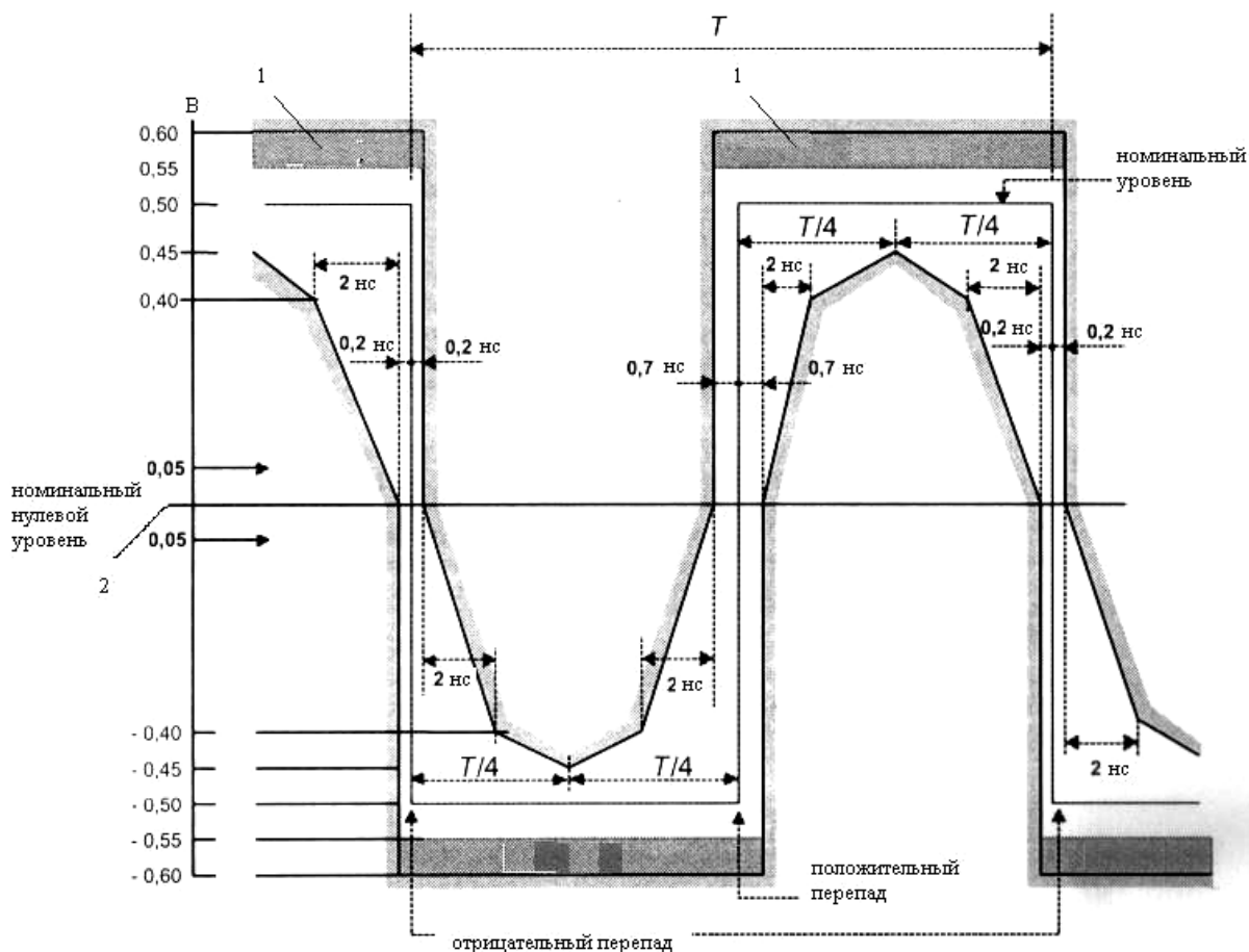
Рисунок 15 - Маска для логической единицы
