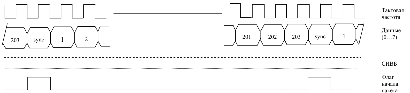
Рисунок 5 – Формат передачи пакетов 204 байт
