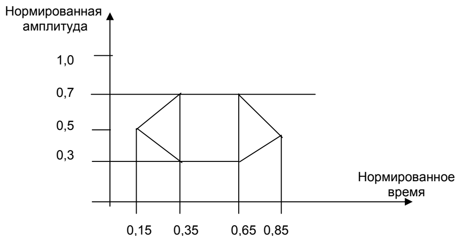
Рисунок 20 - Маска глазковой диаграмма передатчика при измерении джиттера
