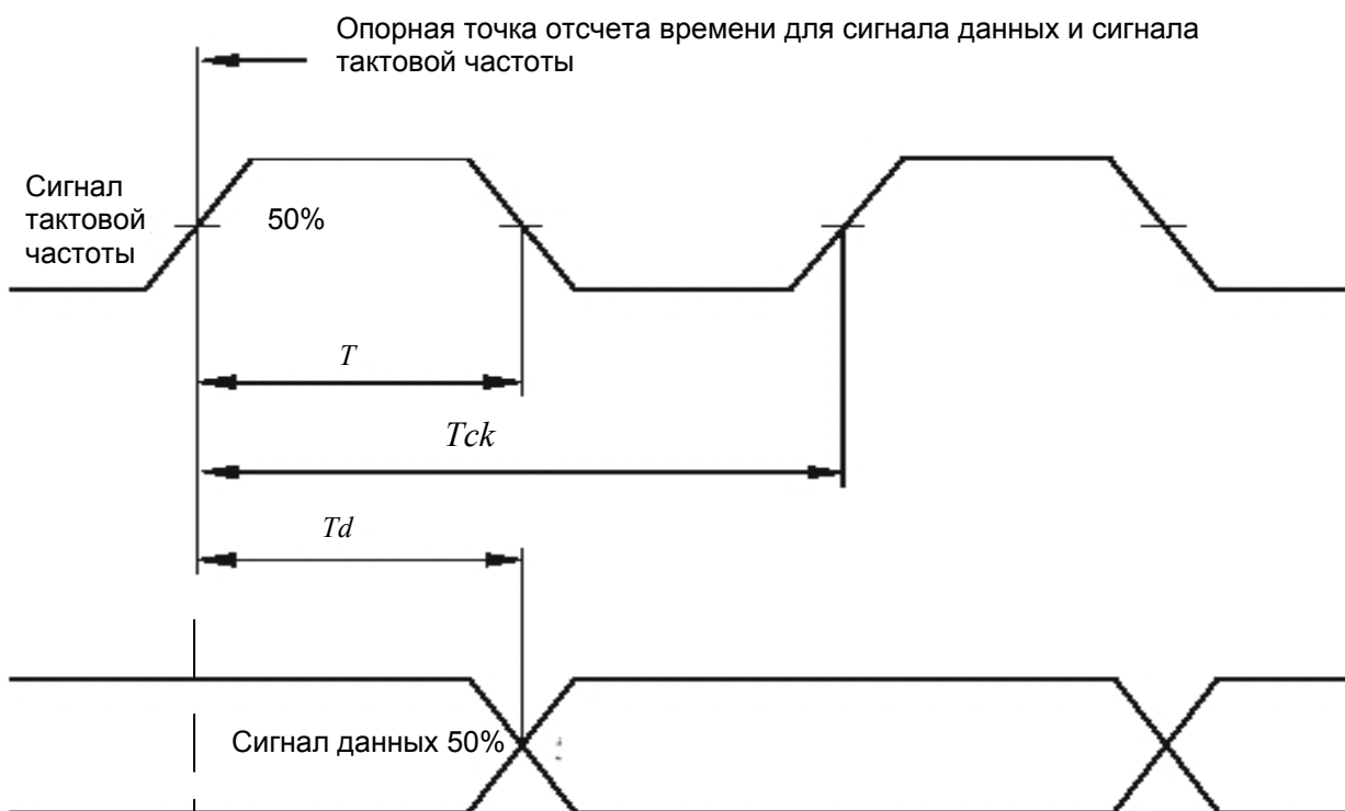
Рисунок 7 - Соотношения параметров синхронизации сигнала и данных
