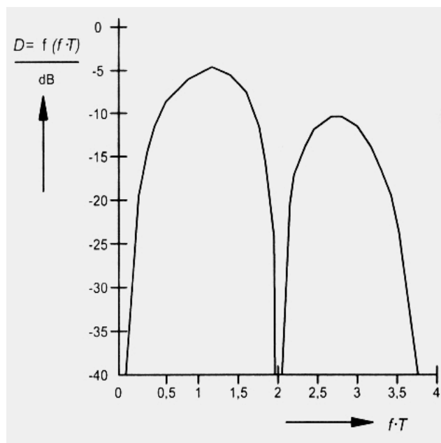
Рисунок 13 - Спектральные плотности инверсного биполярного кода БВН
