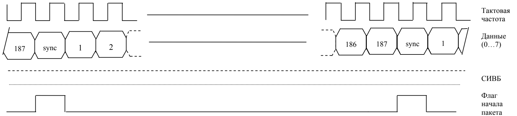
Рисунок 4 – Формат передачи пакетов 188 байт
