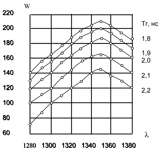
Рисунок 23 - Ширина спектра передатчика
