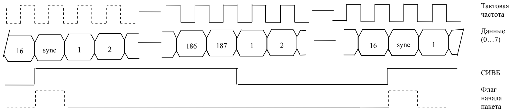
Рисунок 5 – Формат передачи пакетов 204 байт
