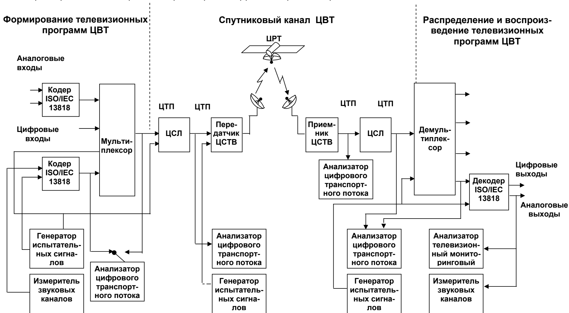
Рисунок Д.1 - Схема измерения параметров цифрового потока в спутниковом канале связи ЦВТ с кодированием и декодированием по стандарту ISO/IEC 13818 [13]
