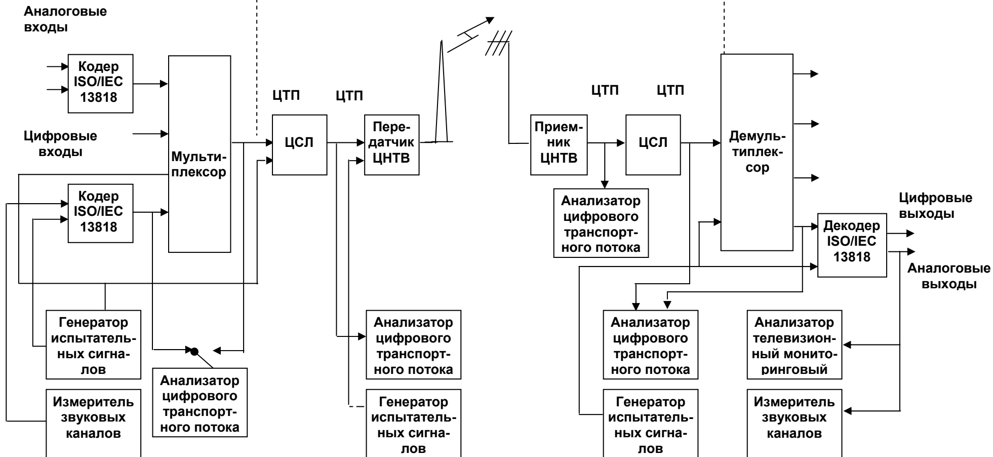
Рисунок Д.2 - Схема измерения параметров цифрового потока в наземном канале связи ЦВТ с кодированием и декодированием по стандарту ISO/IEC 13818
