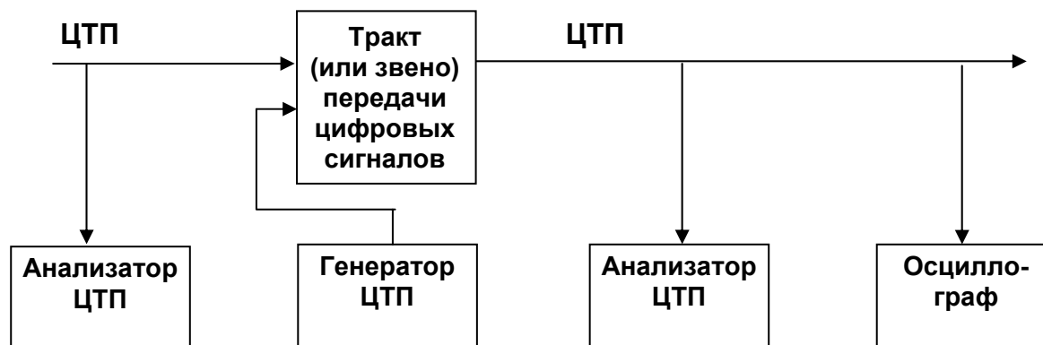
Рисунок 2 - Схема проведения измерений параметров цифрового транспортного потока
