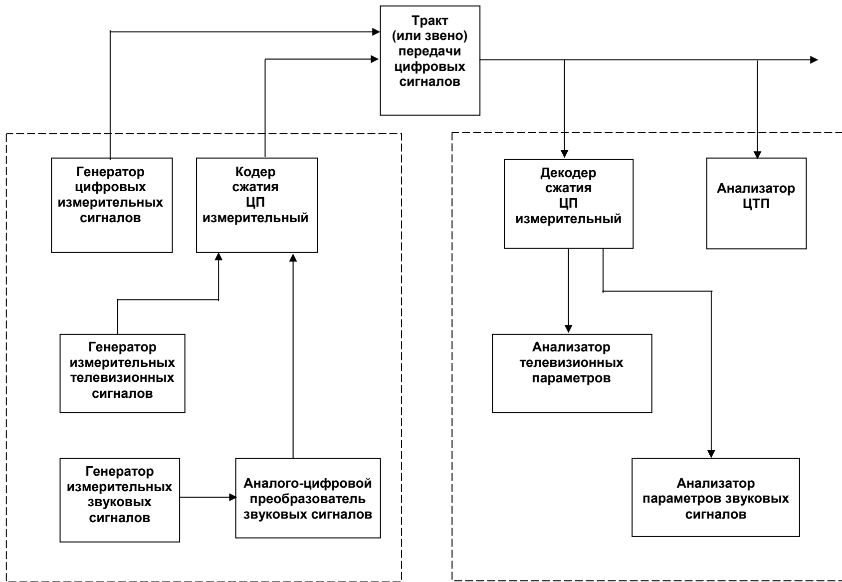
Рисунок 3 - Измерение параметров тракта передачи цифровых сигналов в аналоговом представлении
