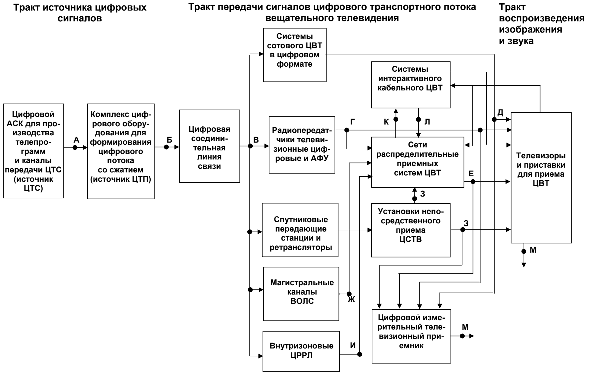
Рисунок 1 - Пример тракта передачи сигналов цифрового вещательного телевидения и его звеньев
