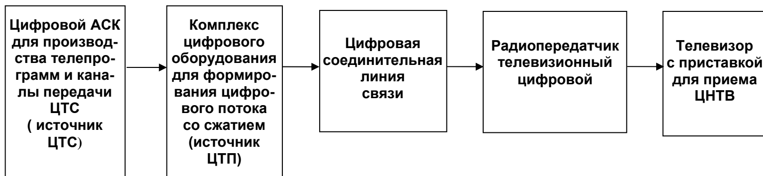
Рисунок Б.1 - Структурная схема типового тракта наземного цифрового телевидения (ЦНТВ)
