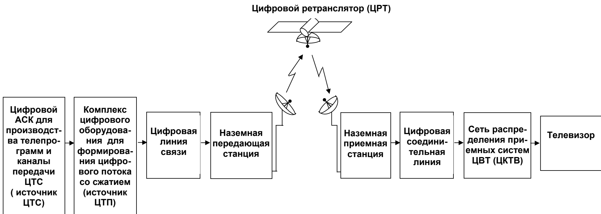
Рисунок Б.4 - Структурная схема типового тракта цифрового спутникового телевидения с ретрансляцией в кабельную сеть
