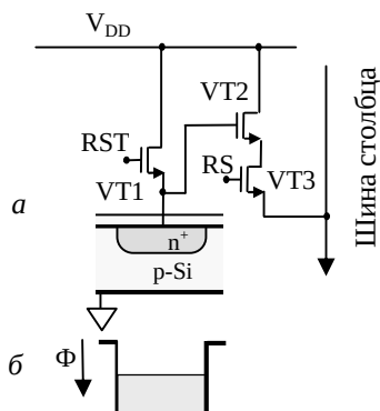
Рис. 1.23. Структура активного пикселя а и соответствующая диаграмма потенциала б
