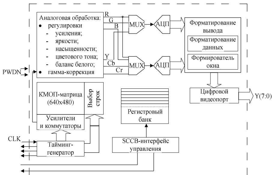
Рис. 4.14. Вideosистема на кристалле OV7640 фирмы OmniVision
