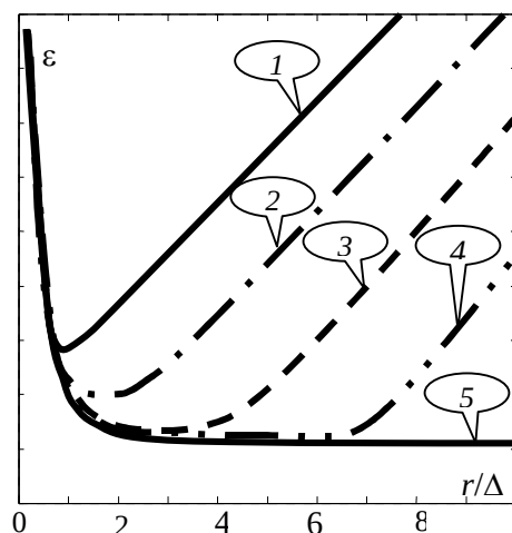
Рис. 2.5. Зависимость относительной ошибки измерения координат сигнала методом центра тяжести при оптимальной дискретизации без фильтрации 1 и при избыточно подробной дискретизации с фильтрацией при числе n членов дискретной двумерной импульсной характеристики:
