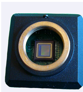
Рис. 1.30. Телекамеры на КМОП фотоприёмниках с внешними устройствами различной сложности от включающей сложные цветковые коррекции (а) до простой (г, справа), содержащей во внешнем устройстве лишь кварцевый генератор (г, слева от КМОП телекамеры)
