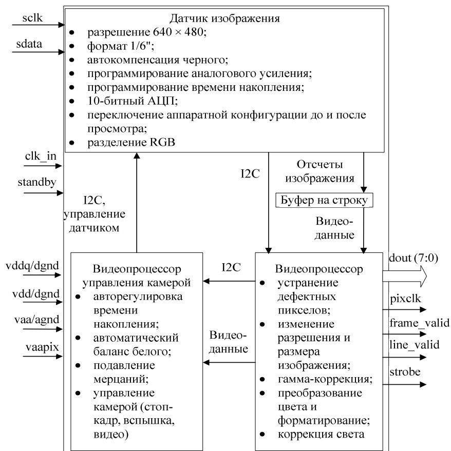
Рис. 4.16. Видеосистема на кристалле MT9V112 фирмы Micron
