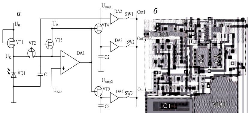
Рис. 1.27. Принципиальная схема а и топология б пиксела с расширенным динамическим диапазоном
