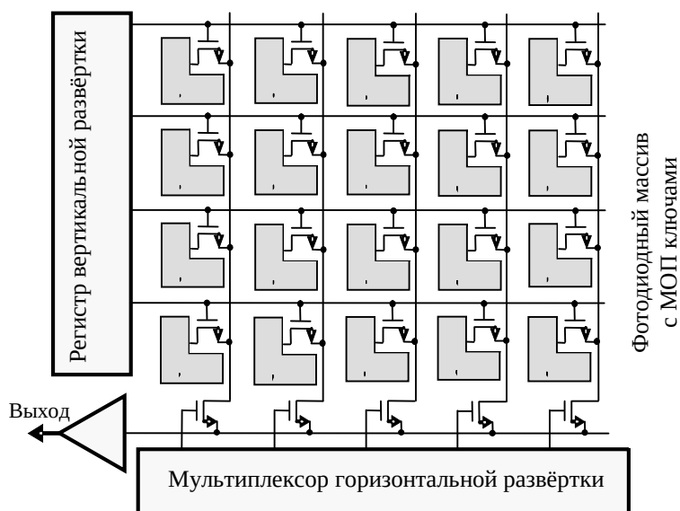
Рис. 1.16. КМОП сенсор с пассивным пикселем
