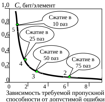
Рис. 4.30 Взаимосвязь требуемой пропускной способности и допустимой среднеквадратической ошибки ( \sigma^2 = \epsilon ) для алгоритма ПРМ при d=4
