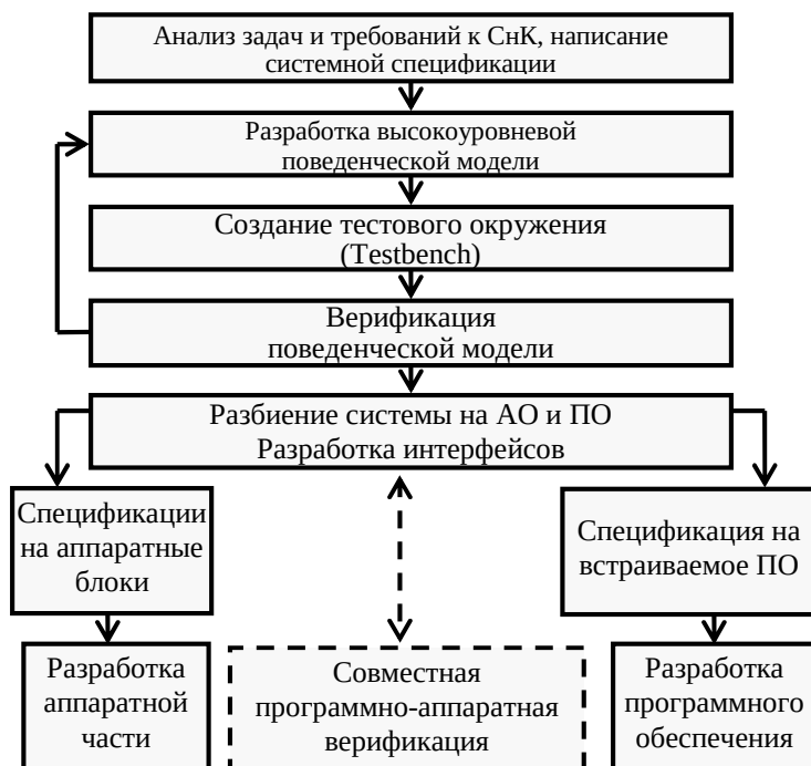
Рис. 4.19. Маршрут концептуального проектирования системы на кристалле
