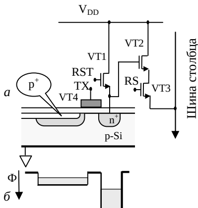
Рис. 1.24. Структура активного пиксела с дополнительным затвором a и соответствующая диаграмма потенциала b
