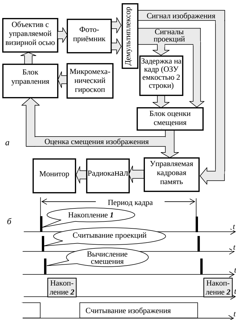
Рис. 2.20. Структурная схема а и временные диаграммы б системы, измеряющей смещение изображений до считывания самого изображения для его стабилизации при наблюдениях с малогабаритных летательных аппаратов
