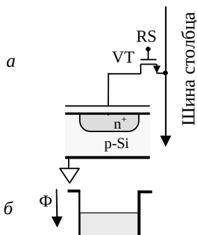
Рис. 1.22. Структура пассивного пикселя а и соответствующая диаграмма потенциала б
