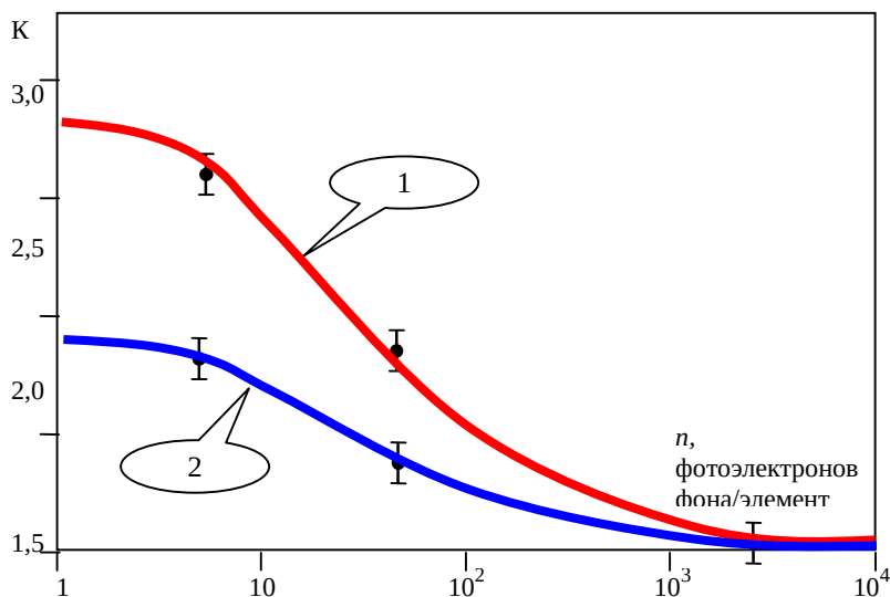
Рис. 2.11. Экспериментальная зависимость выигрыша в чувствительности адаптивной астрономической телекамеры от интенсивности внешнего фона при охлаждении матрицы ПЗС 1 и без охлаждения 2
