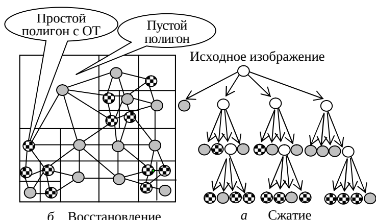
Рис. 4.26. Пирамидальный процесс сжатия и восстановления изображения
