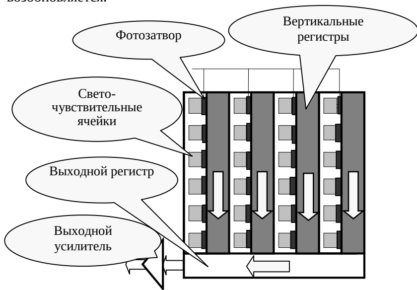
Рис. 1.6. Матричный ПЗС со строчным переносом
