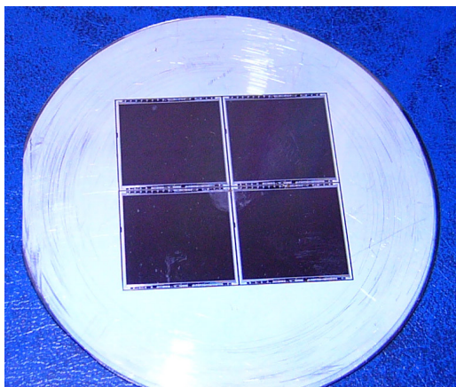
Рис. В.6. Кремниевая пластина диаметром 70 мм с астрономическими матрицами ПЗС класса 1,3 Мегапиксела. Разработки ЦНИИ «Электрон»
