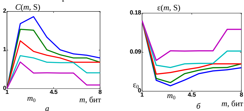
Рис. 3.4. Зависимость пропускной способности a и среднеквадратической ошибки передачи b от разрядности представления базисных функций для сигнала при различных значениях ограничения сложности кодирования S
