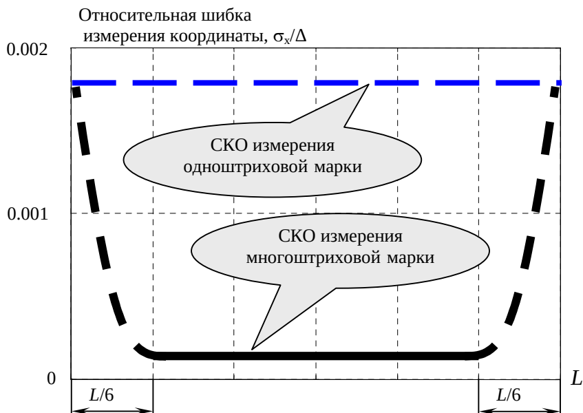
Рис. 2.14. Зависимость ошибки измерения координат многоштриховой метки от ее положения на линейном фотоприёмнике, обусловленная уменьшением числа штрихов на краях поля зрения
