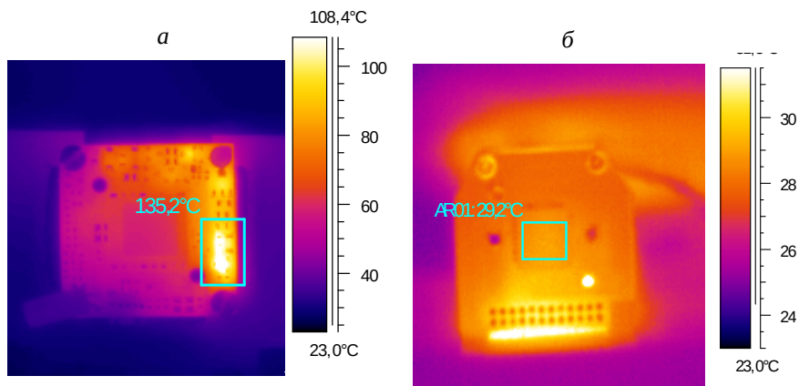
Рис. 1. 32. Распределение температур на матричной плате в телекамере на ПЗС фирмы Sony а и на матричной плате КМОП телекамеры на основе КМОП сенсора фирмы Omni Vision б
