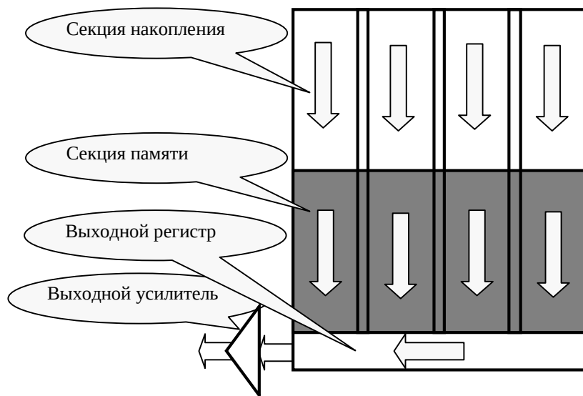
Рис. 1.4. Матричный ПЗС с кадровым переносом
