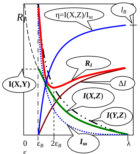
Рис. 3.2. Зависимость информационного риска R_I и его составляющих – потери полезной информации \Delta I и шумовой информации I_{ш} от среднеквадратичной ошибки \epsilon ; минимум информационного риска при равенстве цен потери полезной информации и шумовой информации достигается при полной ошибке \epsilon = 2\epsilon_B , т. е. при коэффициенте шума, равном двум
