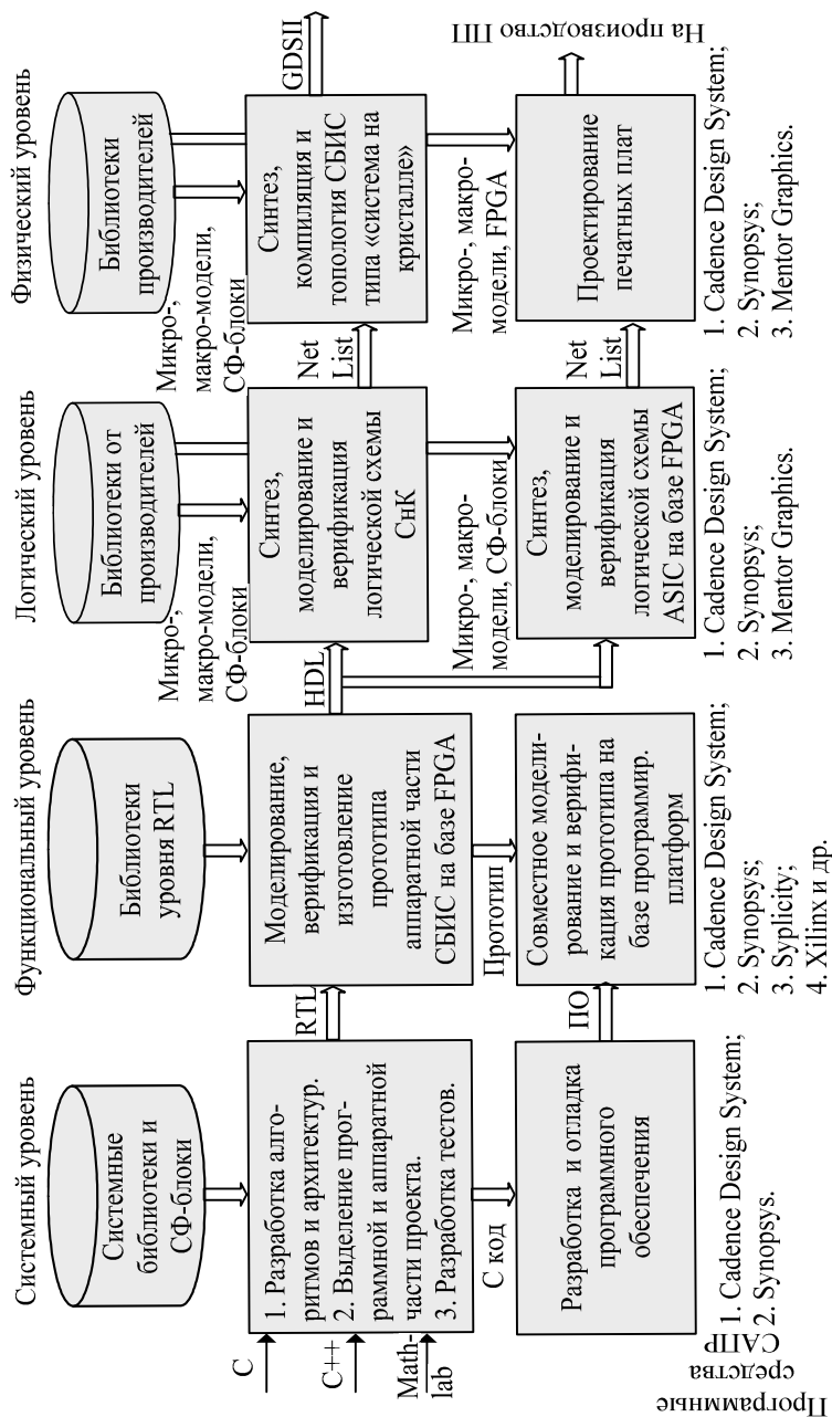
Рис. 4.21. Обобщенный маршрут автоматизированного проектирования СБИС типа «система на кристалле»
