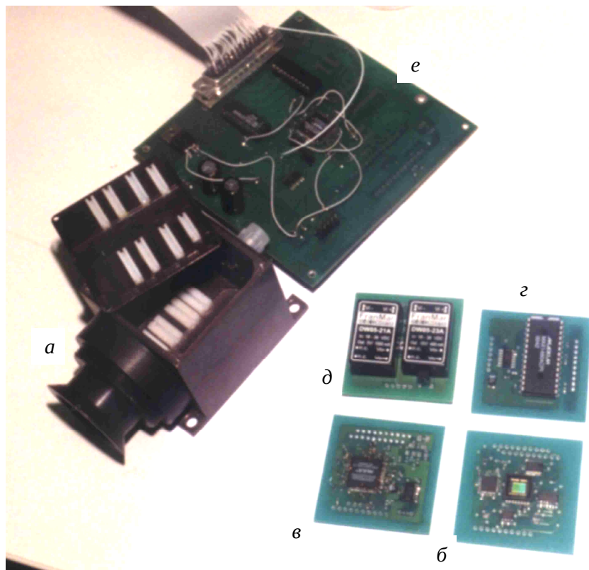
Рис. 1.12. Типовая бортовая телекамера на матричном ПЗС класса 1/4" фирмы Sony; корпус а, плата матрицы ПЗС и видеотракта б, плата синхронизации и адаптации времени накопления от 10^{-4} до 5 с в, плата интерфейса RS-485 г, плата формирователей питающих напряжений телекамеры из бортовой сети 27 В д, плата приёмника-декодера е
