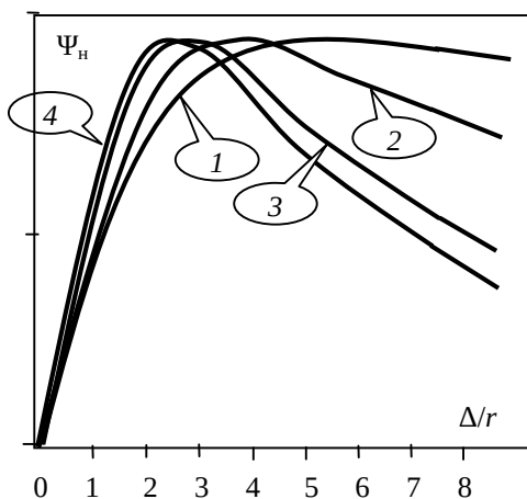
Рис. 2.1. Зависимость нормированного отношения сигнал/шум \Psi_n^2 = \Psi^2 / \Psi_{max}^2 от соотношения размеров элемента разложения и функции рассеяния точки объективом \Delta/r при постоянном уровне полезного сигнала \alpha=100 и шума считывания D=3 и различных значениях фона 1) B=1 , 2) B=10 ; 3) B=100 , 4) B=1000 .
