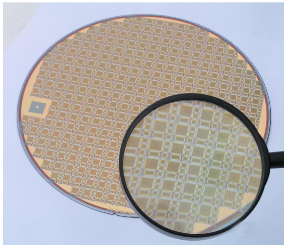
Рис. В.8. Кремниевая пластина диаметром 200 мм с комплектом БИС БПФ разработки «ОТИК дизайн»
