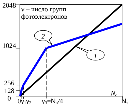
Рис. 3.7. Зависимость числа v групп фотоэлектронов в отсчете с максимальным откликом от интенсивности сигнала N_c (полного числа фотоэлектронов от точечного объекта) при равномерной дискретизации и равномерном квантовании 1 и при адаптивном групповом счете фотоэлектронов 2 при адаптивном счете фотонов для емкости элемента N_3 = 6,4 \times 10^4
