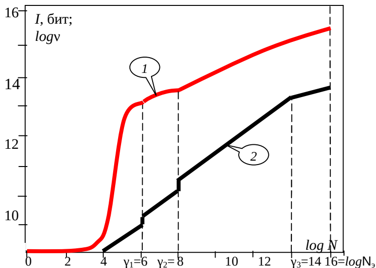
Рис. 3.8. Зависимость количества извлекаемой информации I (по одной из координат) при обнаружении–оценивании координаты точечного объекта для различных вариантов накопления 1, число v групп фотоэлектронов от звезды 2 от количества N сигнальных фотоэлектронов для матрицы с числом элементов на строке 10^3 и накопительной способностью элемента N_3 \approx 64 \times 10^3
