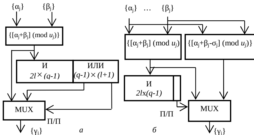
Рис. 3.10. Редуцирование суммы вычетов полной подстановкой
