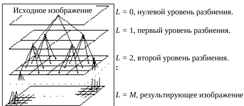
Рис. 4.25. Пирамидальная структура процесса кодирования ПРМ
