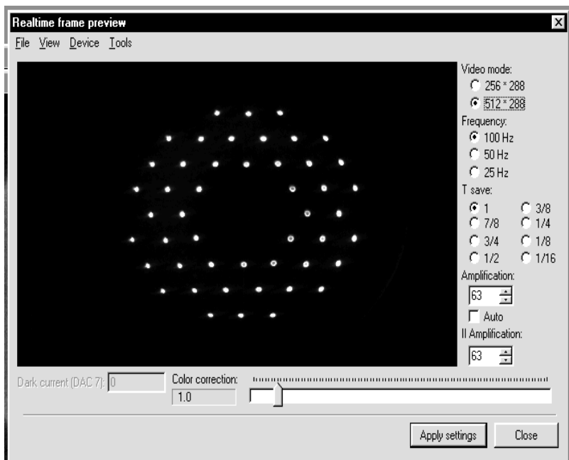
Рис. 2. 12. Изображение гартманограммы и поля управления параметрами твердотельной телекамеры
