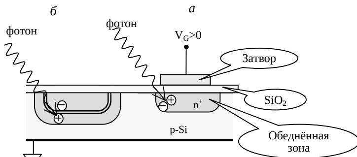
Рис. 1.1. Структура элемента твердотельного фотоприёмника
