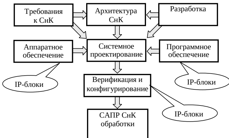
Рис. 4.22 Этапы проектирования СнК обработки изображений
