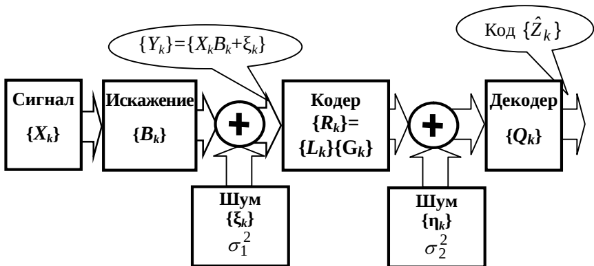
Рис. 3.1. Модель линейного кодирования зашумлённого сигнала
