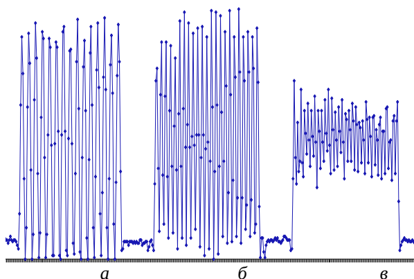
Рис. 2.15. Осциллограммы многоштриховой метки при оптимальном соотношении периода метки и шага дискретизации a , при несколько меньшем периоде, когда количество информации о координате метки уменьшается из-за корреляции ошибок измерения координат максимумов и минимумов б , и при существенно меньшем периоде метки, когда количество информации о координате метки уменьшается из-за уменьшения глубины модуляции сигнала метки в
