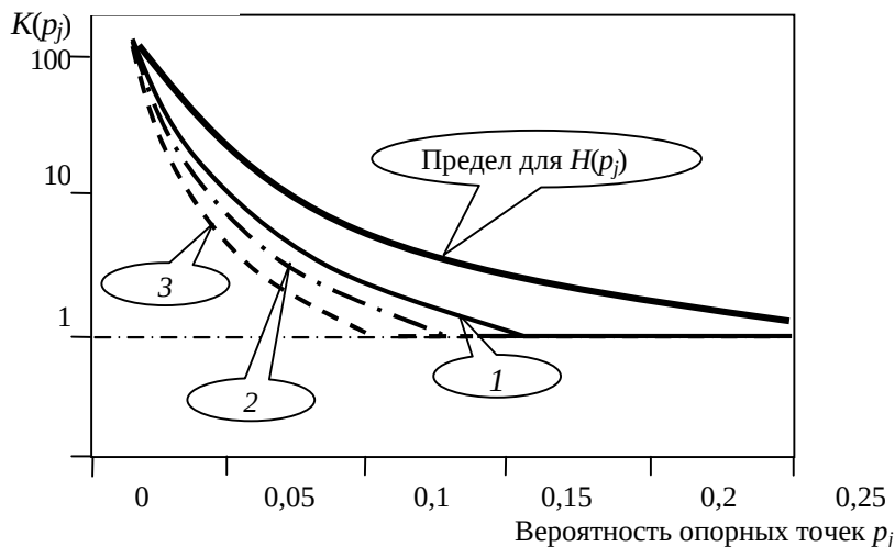
Рис. 4.29. Зависимость коэффициента сжатия от числа опорных точек при различных видах разбиения d=3 1, d=4 2, d=6 и d=2 3
