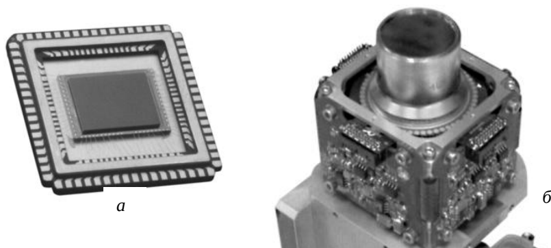
Рис. 1.36. ИК матрица а и матричный блок с ней с электронными платами и германиевым входным окном б
