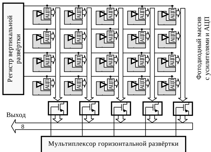
Рис. 1.21. КМОП сенсор с активным цифровым пикселем
