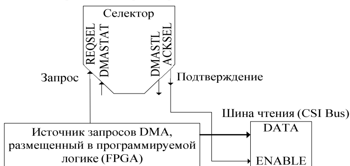
Рис. 4.8. Структура селектора DMA при записи в память
