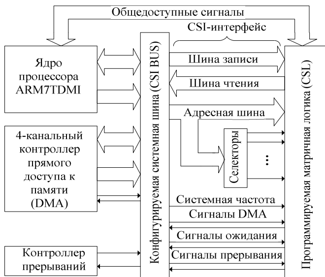
Рис. 4.8. Конфигурируемая системная шина и ее окружение
