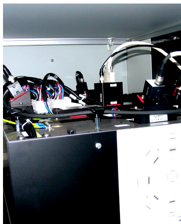
Рис. 4.3. Многоракурсная телевизионно-компьютерная система контроля печатных узлов (вид изнутри)
