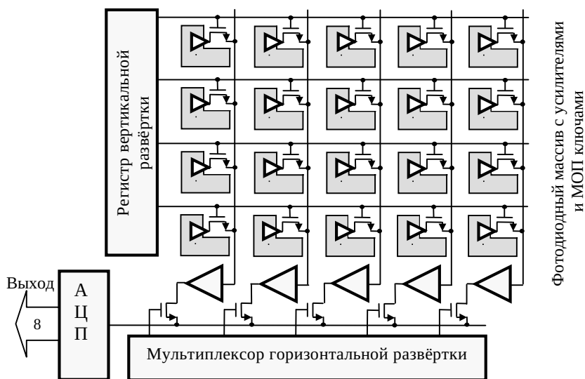
Рис. 1.19. КМОП сенсор с активным пикселом, активным столбцом и одним АЦП
