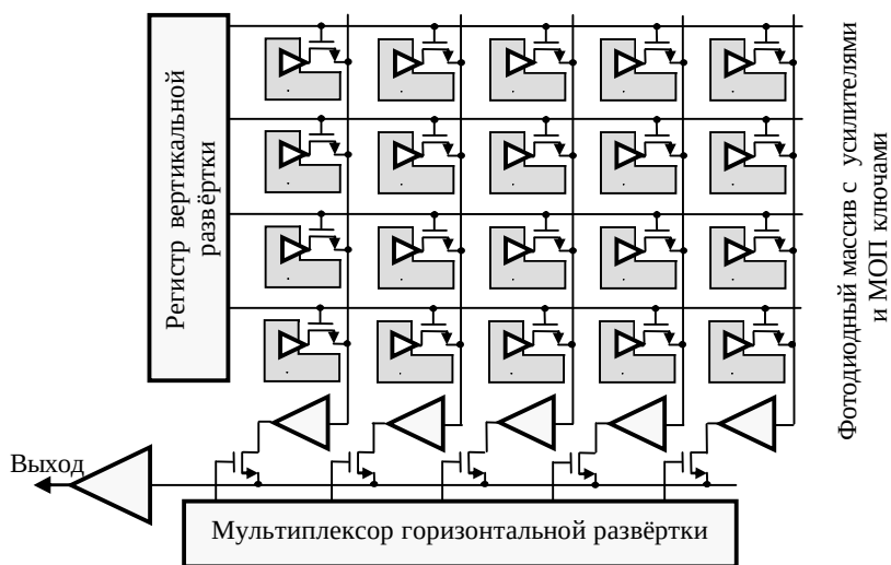
Рис. 1.18. КМОП сенсор с активным пикселом и активным столбцом
