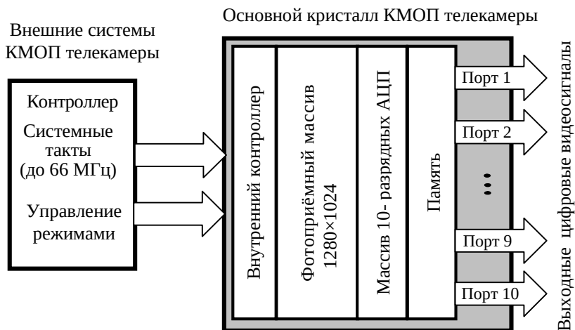
Рис. 1. 29. Структура КМОП сенсора MT9M413 фирмы Micron с активным пикселем и АЦП на каждый столбец, размещаемой в 280-выводном керамическом корпусе
