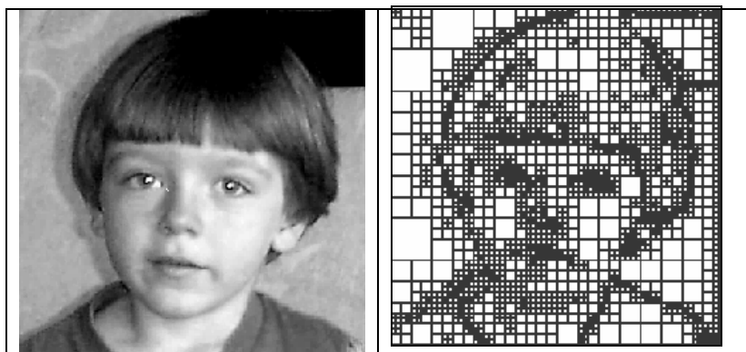
Рис. 4.31. Иллюстрация работы алгоритма ПРМ при разбиении на каждом уровне кодирования априорного интервала на 4 части ( d = 4 )
