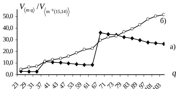
Рис. 3.13. Отношение аппаратной сложности таблично реализованных каналов \langle m q \rangle и двухступенчатых каналов \langle m^q(15,14) \rangle :
