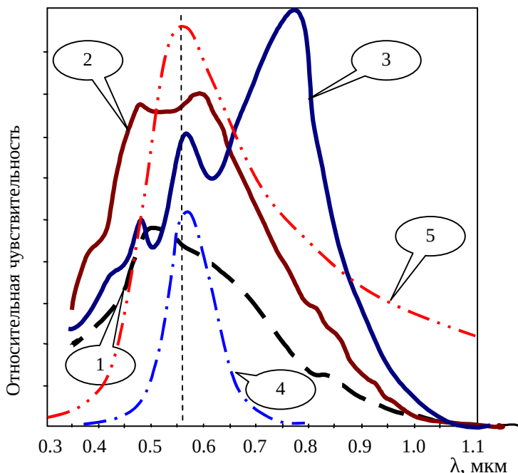
Рис. 1.8. Спектральные характеристики чувствительности ПЗС: 1 – со строчным переносом, 2 – Exview ПЗС, 3 – ПЗС с кадровым переносом; для сравнения приведены спектральная характеристика зрения 4 и спектральная характеристика излучения абсолютно чёрного тела с температурой 6000К, которая служит огибающей спектра излучения Солнца 5
