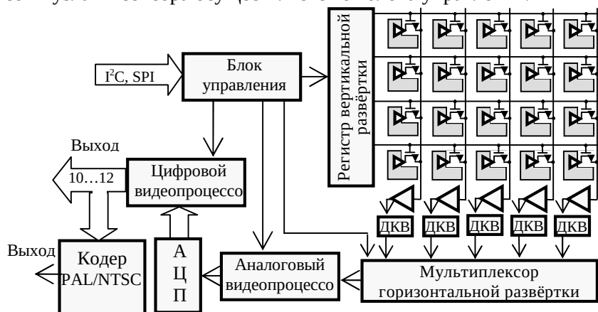
Рис. 1.28. Типовая структура КМОП сенсора с активным пикселем, активным столбцом, аналоговым и цифровым процессором
