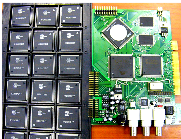
Рис. 4.1 Система на кристалле: декодер MPEG-2; топология а и партия СБИС с платой прототипа б
