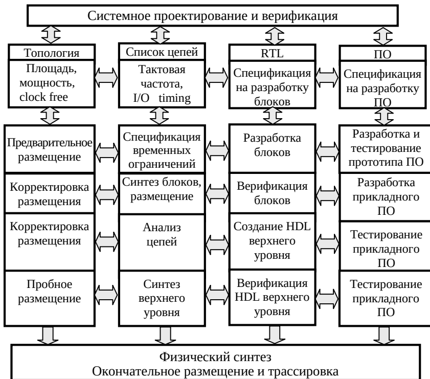
Рис. 4.18. Спиралевидная модель процесса проектирования с использованием технологии «система на кристалле»
