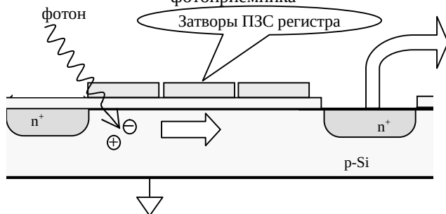
Рис. 1.2. Структура считывания сигнала в твердотельном фотоприёмнике
