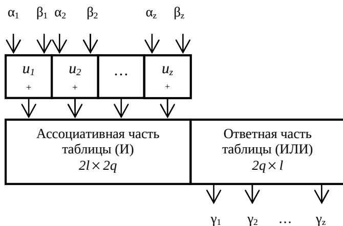
Рис. 3.10. Редуцирование суммы вычетов полной подстановкой
