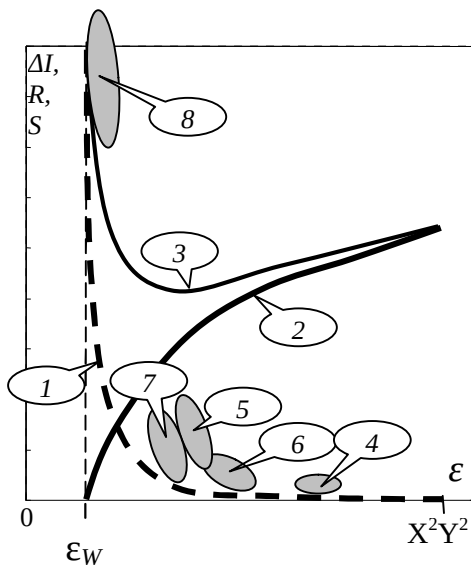
Рис. 2.4. Взаимосвязь сложности и точности измерения координат.
