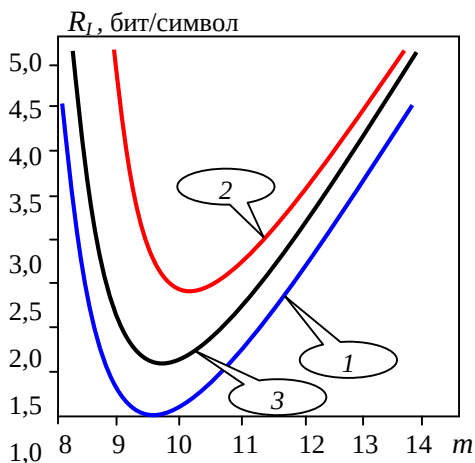
Рис. 3.6. Зависимость информационного риска от числа разрядов при неравномерном квантовании с непрерывно изменяющимся шагом (1), равномерном квантовании (2), и двухчастотном квантовании с шагом квантования первой четверти диапазона в четыре раза меньшим, чем в остальной части диапазона амплитуд сигналов (3) для ёмкости элемента разложения N_e \approx 6 \cdot 10^4 электронов
