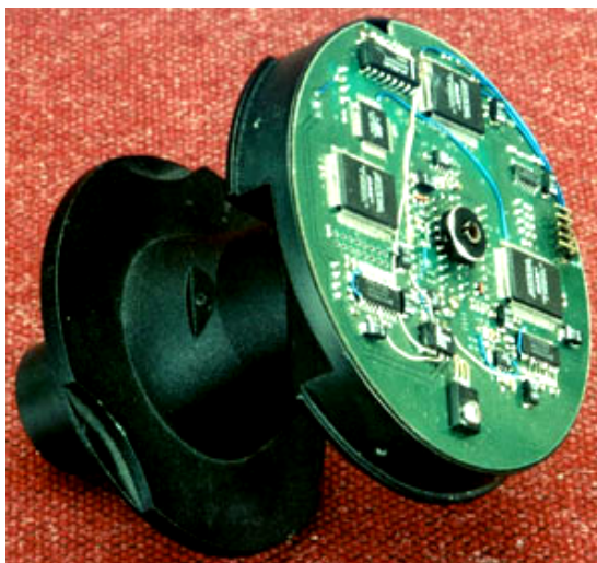
Рис. 2.13. Оптико-электронный преобразователь гравиметрического датчика на двух линейных ПЗС фирмы Sony разработки ЦНИИ «Электроприбор»
