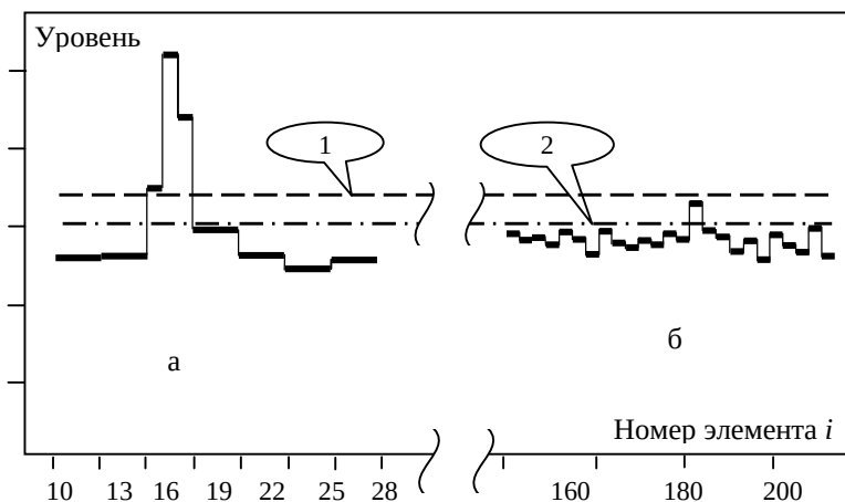
Рис. 2.10. Осциллограммы сигнала при адаптивной дискретизации. Интервал дискретизации для слабых сигналов, не превышающих порог 1, в три раза больше, чем для интенсивных сигналов a ; слабый сигнал, не превышающий порог 1 при подробной дискретизации, превышает порог 2 и обнаруживается при адаптивной дискретизации, б
