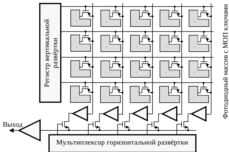
Рис. 1.17. КМОП сенсор с пассивным пикселом и активным столбцом
