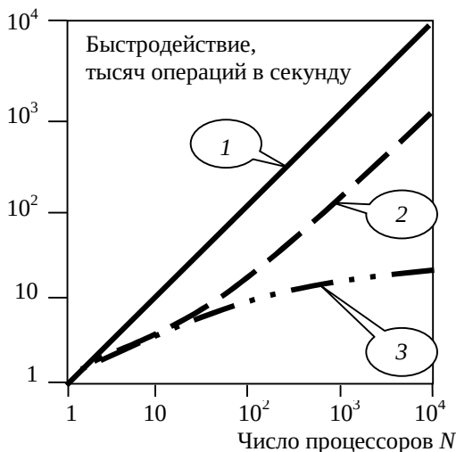
Рис. 4.5. Зависимость увеличения быстродействия, обеспечиваемого одновременно работающими N процессорами.
