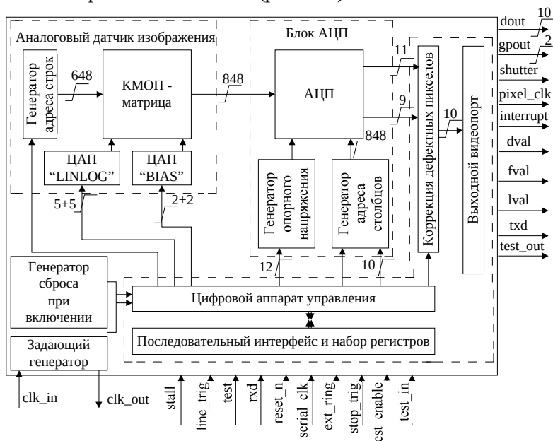
Рис. 4.17. Видеосистема на кристалле ZDM33220 фирмы ZMD AG
