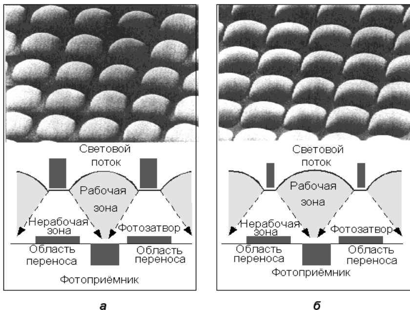
Рис. 1.7. Структура матриц ПЗС: а – стандартная, б – Hyper-HAD
