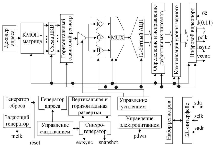
Рис. 4.15. Видеосистема на кристалле КАС-9628 фирмы Kodak
