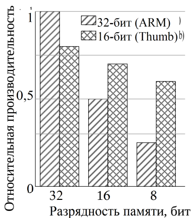
Рис. 4.7. Производительность ядра
