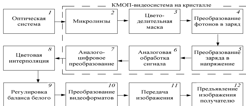
Рис. 4.12. Видеосистема на кристалле в типовой телевизионной системе
