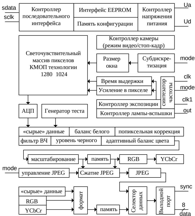
Рис. 1.31. Структура видеосистемы на кристалле ADCC-3960 фирмы Avago Technologies, построенной на основе 1,3-мегапиксельного КМОП датчика изображения
