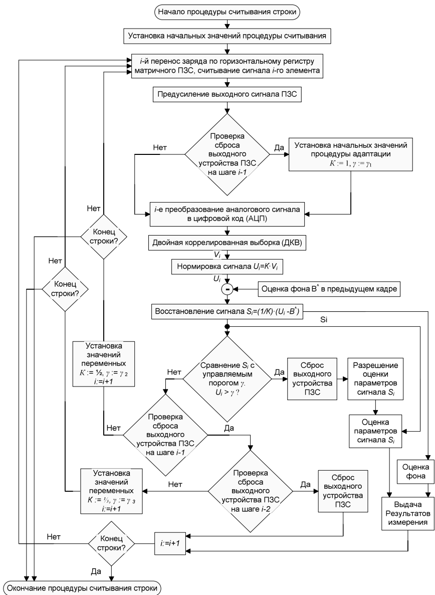
Рис. 2.8. Алгоритм адаптации размера элемента разложения матричного ПЗС к значению накопленного заряда
