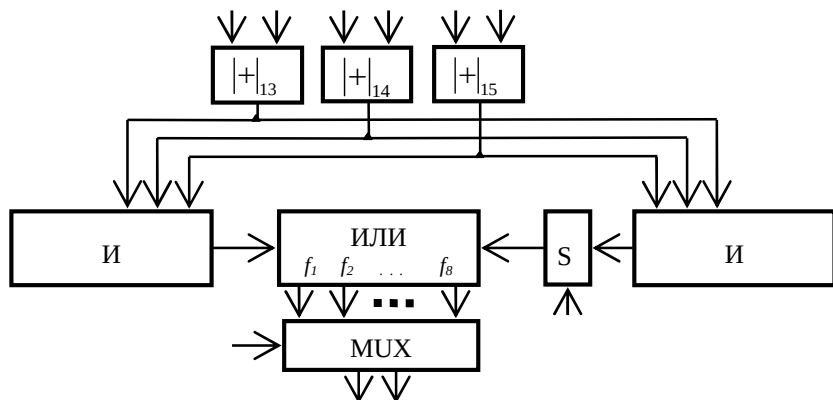
Рис. 3.12. Канал \langle m^q(15,14,\dots) \rangle двухступенчатой МВС с реструктуризированной ассоциативной таблицей
