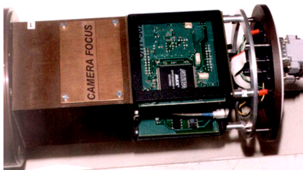
Рис. 1.11. Телекамера для астрономических применений в составе скоростного датчика волнового фронта (кадровая частота до 200Гц); матрицы ПЗС класса \frac{1}{2} " фирмы Sony
