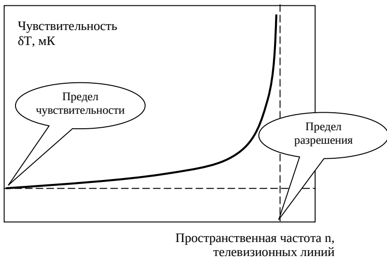
Рис. 1. 34. Зависимость эквивалентной шуму разницы температур от пространственной частоты
