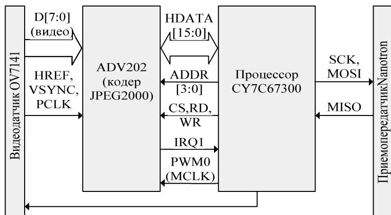
Рис. 4.35. Структурная схема беспроводной видеокамеры
