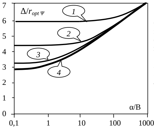
Рис. 2.2. Зависимость оптимального размера элемента разложения при обнаружении от потенциального контраста : 1) B=10 , D=1000 ; 2) B=10 , D=100 ; 3) B=10 , D=10 ; 4) B=10 , D=1 ;
