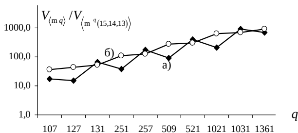
Рис. 3.14. Отношение аппаратной сложности таблично реализованных каналов \langle m q \rangle и двухступенчатых каналов \langle m^q(15,14,13) \rangle :
