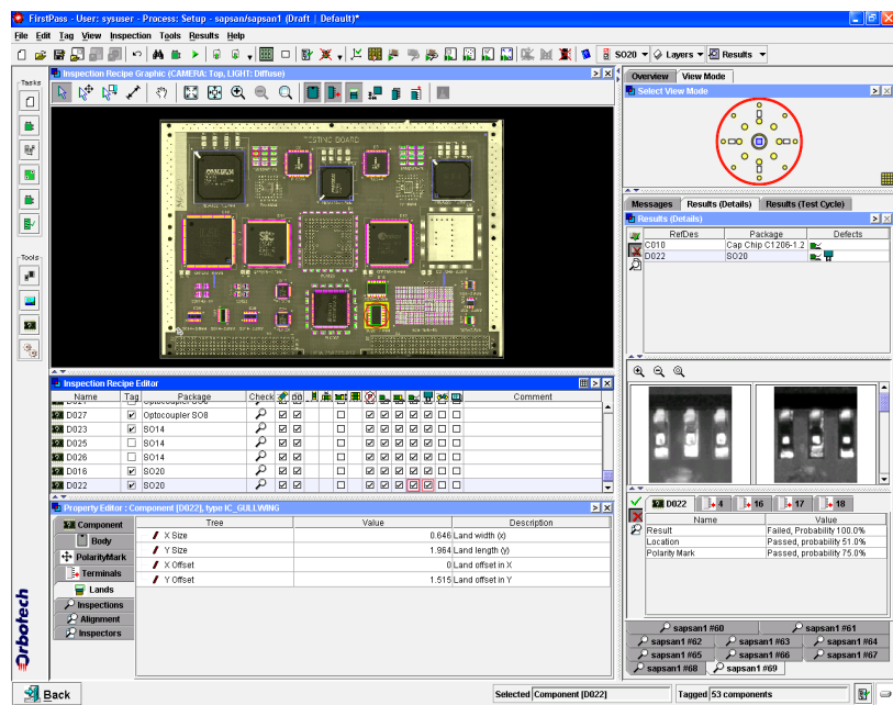
Рис. 4.4. Вид экрана монитора телевизионно-компьютерной системы контроля качества печатных плат.
