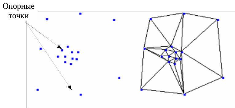
Рис. 4.24. Триангуляция опорных точек изображения
