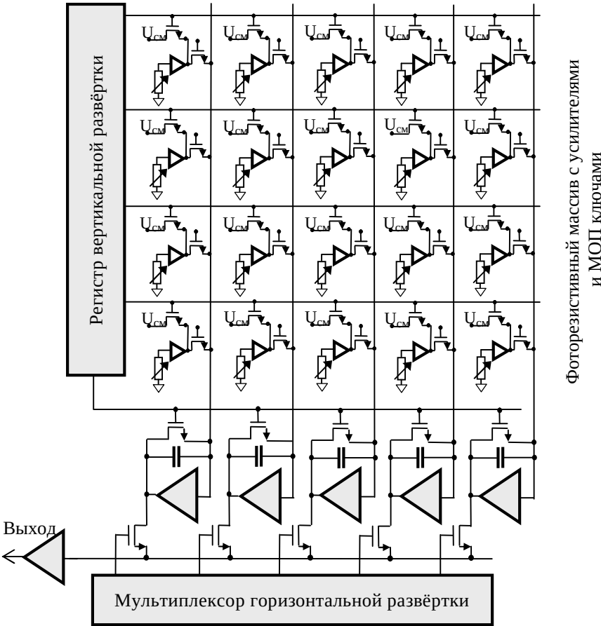
Рис. 1.35. Микроболометрическая матрица для дальнего ИК диапазона с КМОП мультиплексорами
