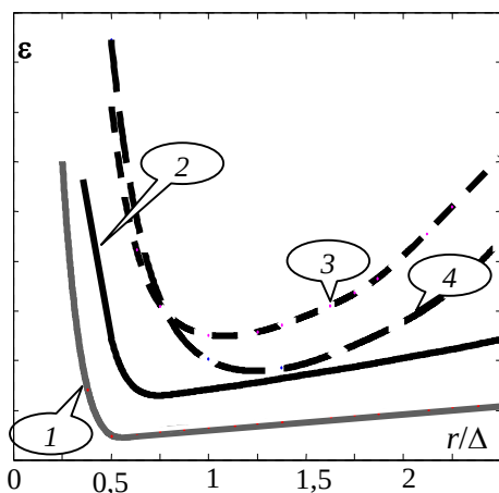
Рис. 2.3. Зависимость относительной ошибки \varepsilon измерения координат сигнала гауссовской формы при аддитивном шуме для различных алгоритмов:
