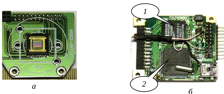
Рис. 4.34. Платы видеокамеры на основе КМОП фотоприёмной матрицы а, кодера источника JPEG2000 б и радиоинтерфейса Wi-Fi в
