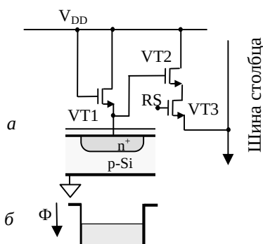
Рис. 1.26. Структура активного пиксела с логарифмической шкалой а , и соответствующая диаграмма потенциала б
