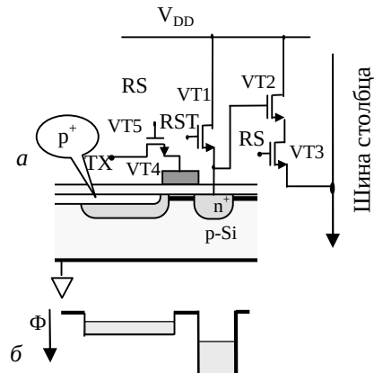
Рис. 1.25. Структура активного пиксела с дополнительным затвором и усилителем в цепи затвора a и соответствующая диаграмма потенциала b
