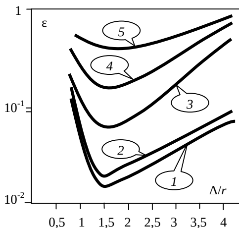
Рис. 2.7. Зависимость среднеквадратической ошибки измерения координат звезды от соотношения размеров элемента разложения и функции рассеяния точки объективом при различных соотношениях шума фона и собственного шума телекамеры 1) \alpha=100, B=5, D=5 ; 2) \alpha=100, B=5, D=10 ; 3) \alpha=100, B=50, D=5 ; 4) \alpha=100, B=100, D=5 ; 5) \alpha=10, B=1, D=1 .
